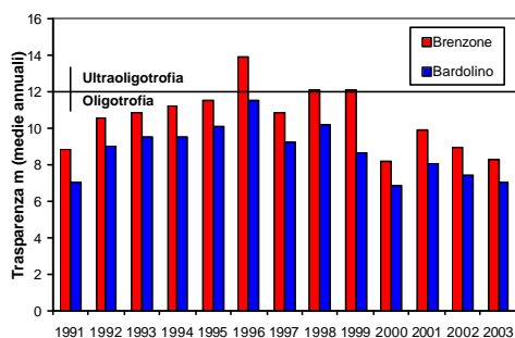
Figura 4: Andamento temporale dei valori medi annuali di trasparenza misurati nelle stazioni di Brenzone e Bardolino. Per la valutazione dello stato trofico (ultraoligotrofia, oligotrofia, mesotrofia) sono riportati i livelli previsti dall'O.E.C.D. – 1982 (Fonte: Salmaso N. (Università degli Studi di Padova), Decet F.(ARPAV Dipartimento Provinciale di Belluno), Franzini G. (ARPAV Dipartimento Provinciale di Verona), Cordella P. (Università degli Studi di Padova); 2001 – AIOL – Associazione Italiana Oceanologia Limnologia, 14:109-123; aggiornato e modificato da ARPAV – Dipartimento Provinciale di Verona)
