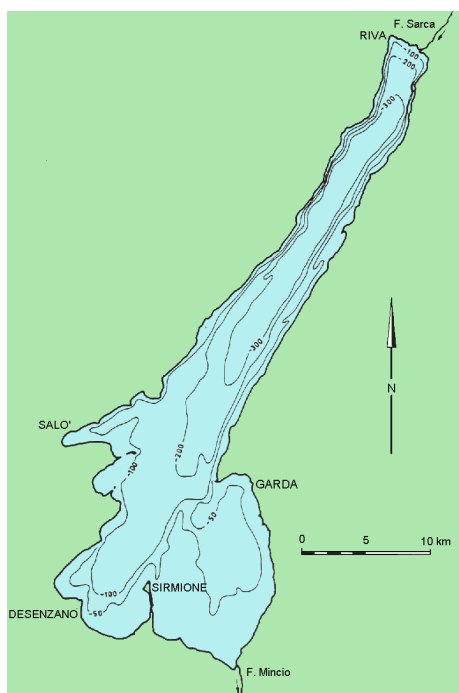
Figura 1: Mappa batimetrica del lago di Garda (CNR, 2004)
